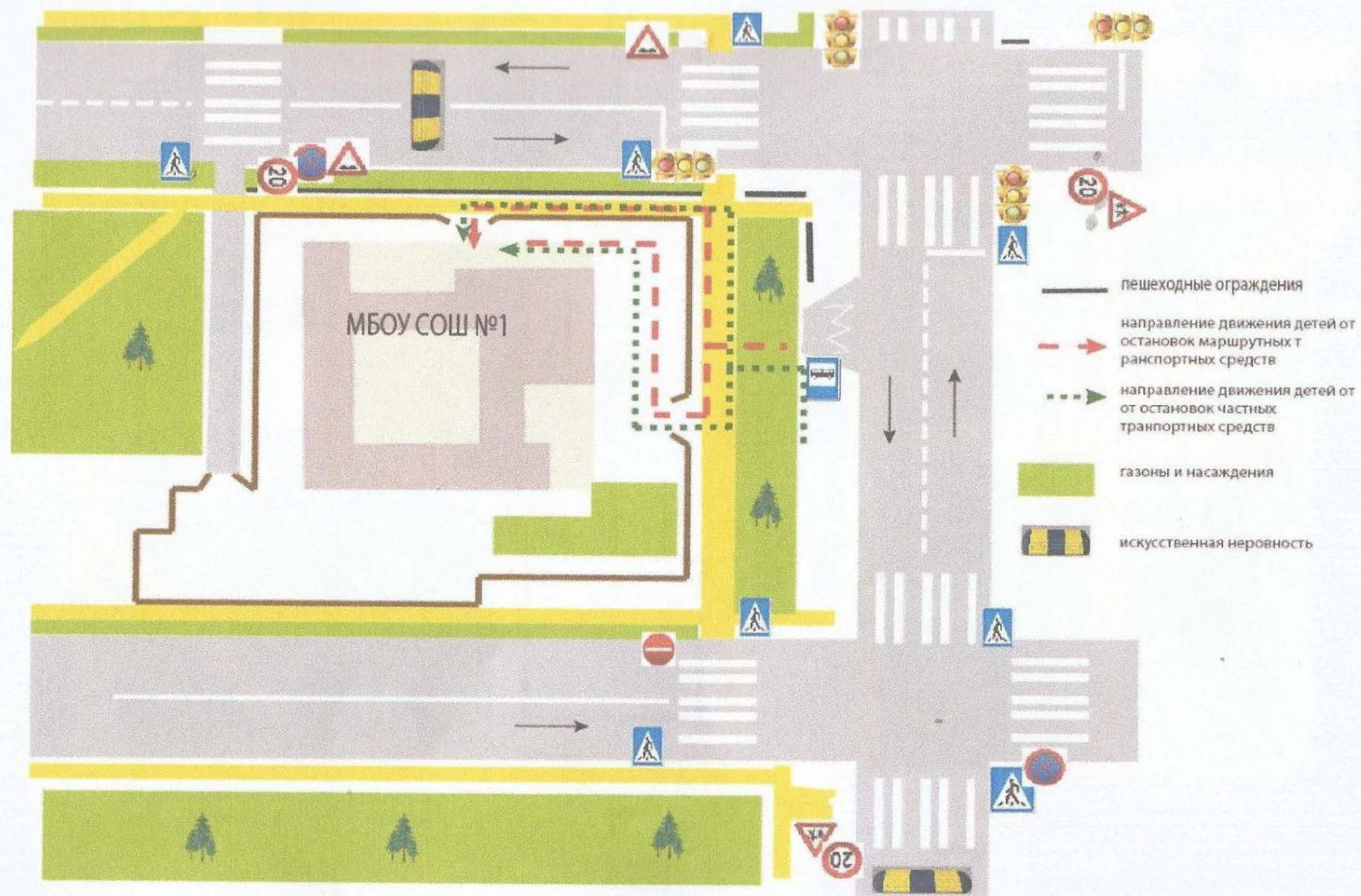
Схема организации дорожного движения в непосредственной близости от образовательного учреждения с размещением соответствующих технических средств, маршруты движения детей от остановок маршрутных транспортных средств, маршруты движения детей от остановок частных транспортных средств
